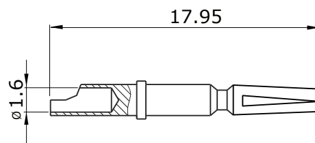
Hauptabmessungen Kontaktbuchse
