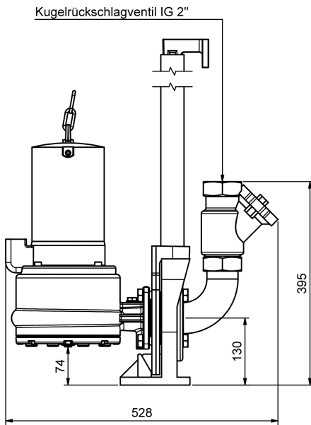
Stationäre Aufstellung
