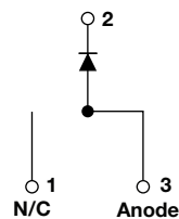
D²PAK (TO-263AB)
