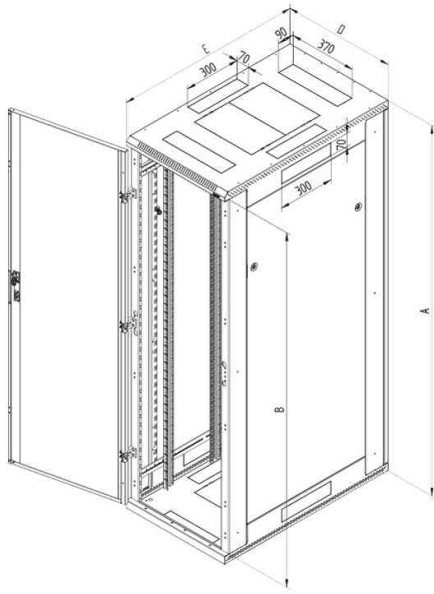
Symbolzeichnung: 19" Netzwerkschrank RJA, einfache Glastür geöffnet (Abbildung ähnlich)
