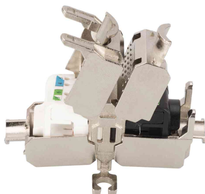
Kat.6A Verbinder, offen
