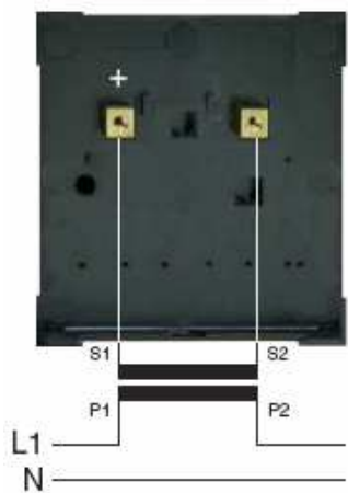
Eingang .../5A oder .../1A AC
