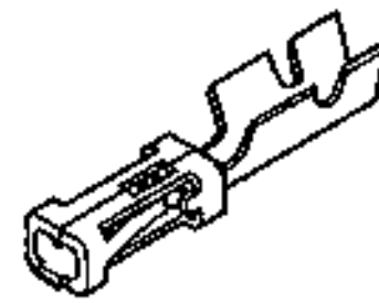
TE Teilenummer 167021-2 MOD-4 REC.CONT.SCP.
