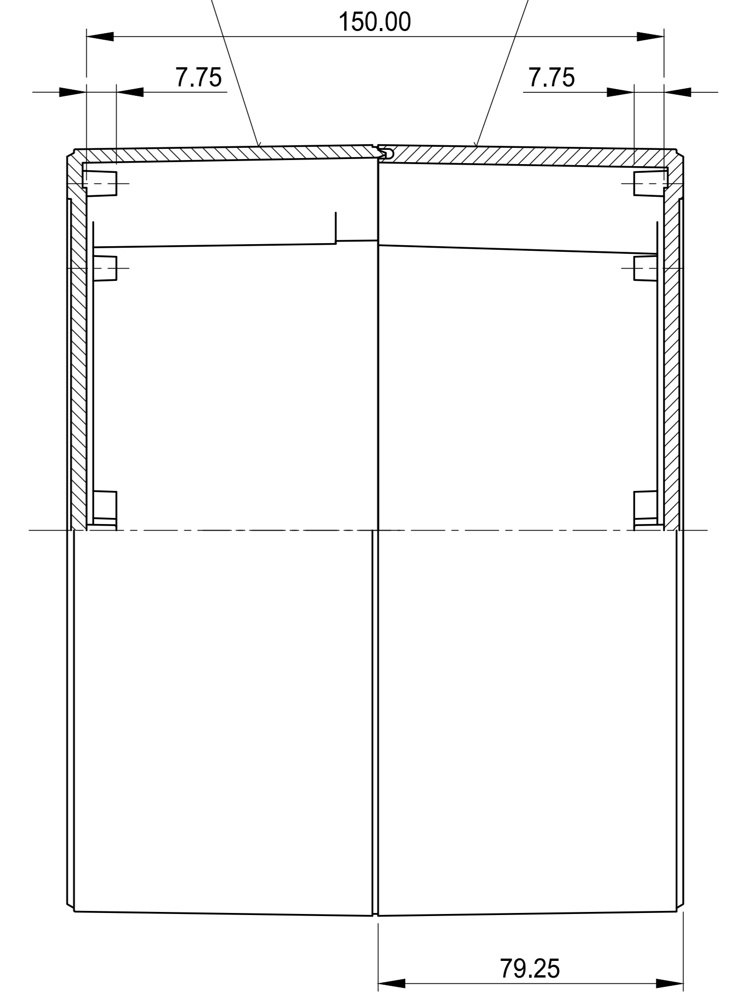
Schnitt B-B section
