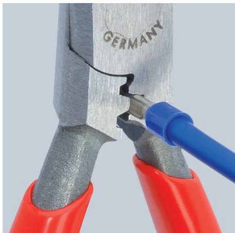
Krimpelés 0,5 - 2,5 mm 2
