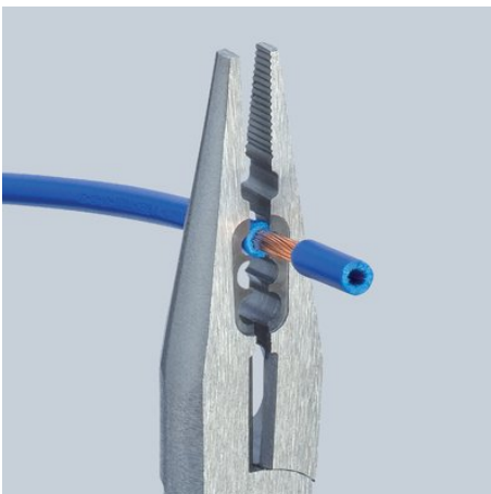
Csupaszítás
