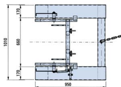
Draufsicht MT 240 Maße in mm
