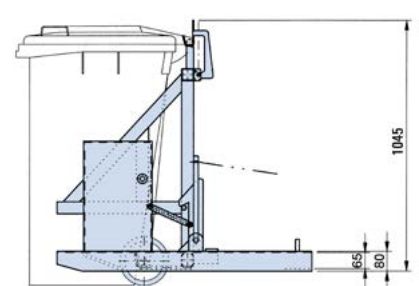
Seitenansicht MT 240 Maße in mm
