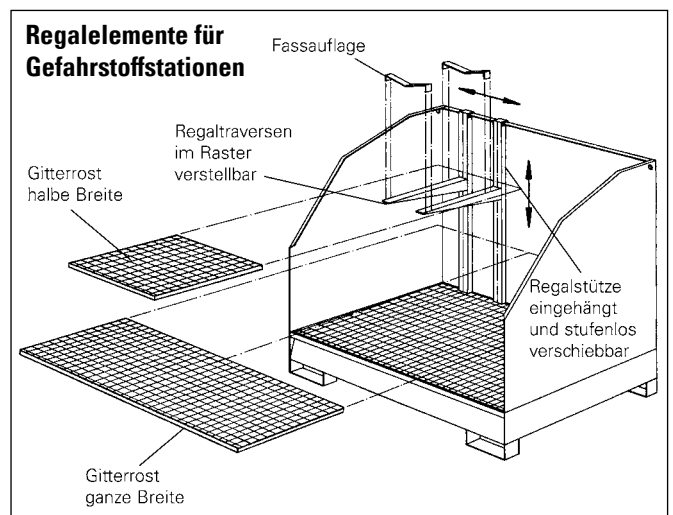
Gefahrstoffdepot Typ 4 GST-K, lackiert, mit Regal für 2 Fässer à 60 Liter
