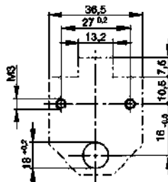
Montageausschnitt
