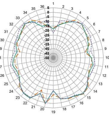
XZ-Plane Gain
