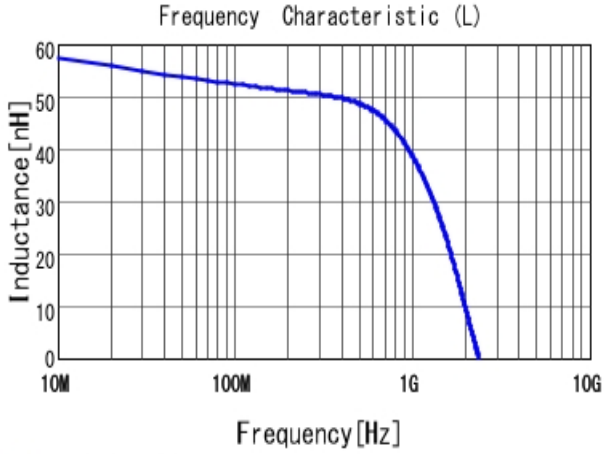
■ LQW18CA56NJ00 L
