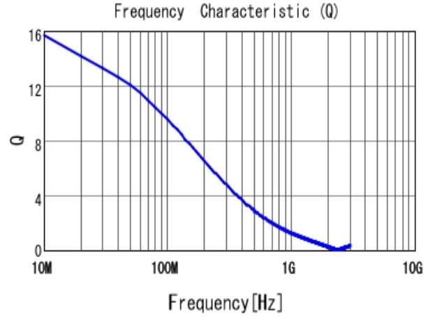
■ LQW18CA56NJ00 Q
