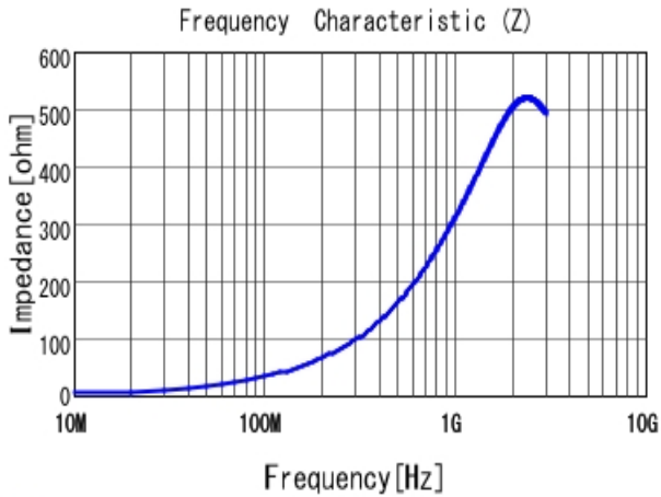
■ LQW18CA56NJ00 |Z|
