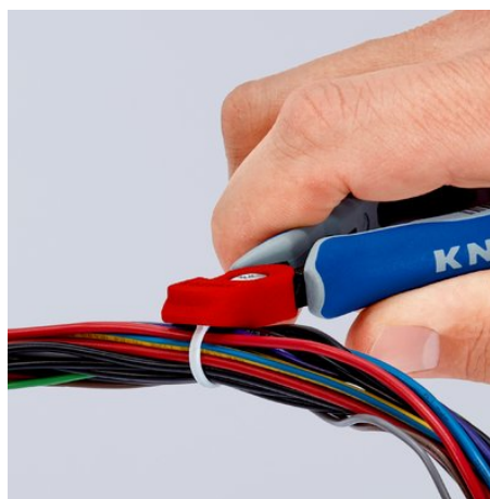
Retirez la bride du collier à l'aide de la pince coupante de côté pour l'électronique...
