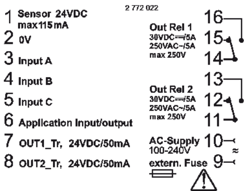
VAC Schaltnetzteil 2 Relais / 2 Transistoren
