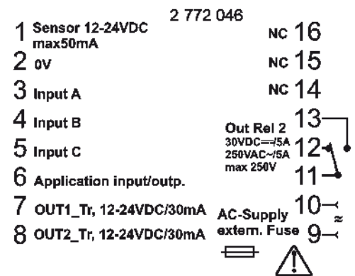
VAC Trafo 1 Relais / 2 Transistoren
