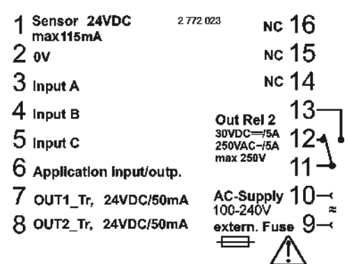
VAC Schaltnetzteil 1 Relais / 2 Transistoren
