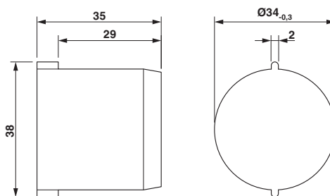
Maßzeichnung
