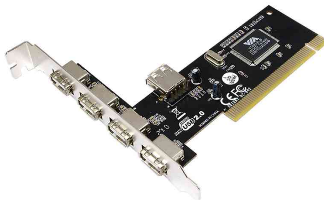
USB 2.0 PCI Karte, 4 + 1 Port - VIA Chipsatz
