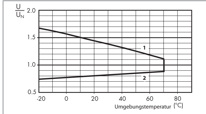
R 46 - AC Spulen-Betriebsspannungsbereich
