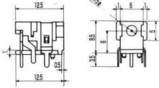
No.M05-532A0 DC JACK FOR P.C.B. (center hole : 1.45 φ mm) JSBJ 5 (DC 13.5V ~18V)
