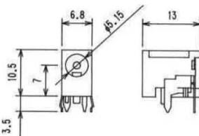
No.M04-754A0 DC JACK FOR P.C.B. (center pin : 1.65 φ mm I.D. : 5.15 φ mm) JSAJ 3 (DC 6.3V ~10.5V)
