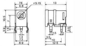
No.MJ-18 (center hole : 1.05 φ mm I.D. : 5.15 φ mm) JSAJ 3 (DC 6.3V ~10.5V)
