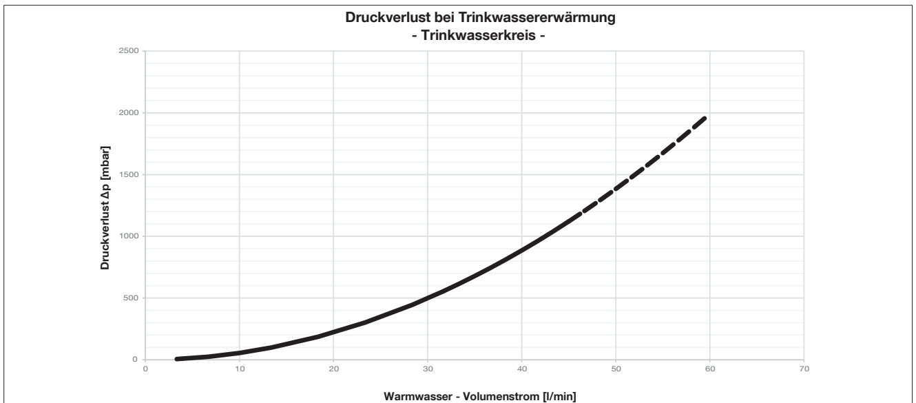
Abb. 5: Kennlinie Druckverlust bei Trinkwassererwärmung (Trinkwasserkreis)
