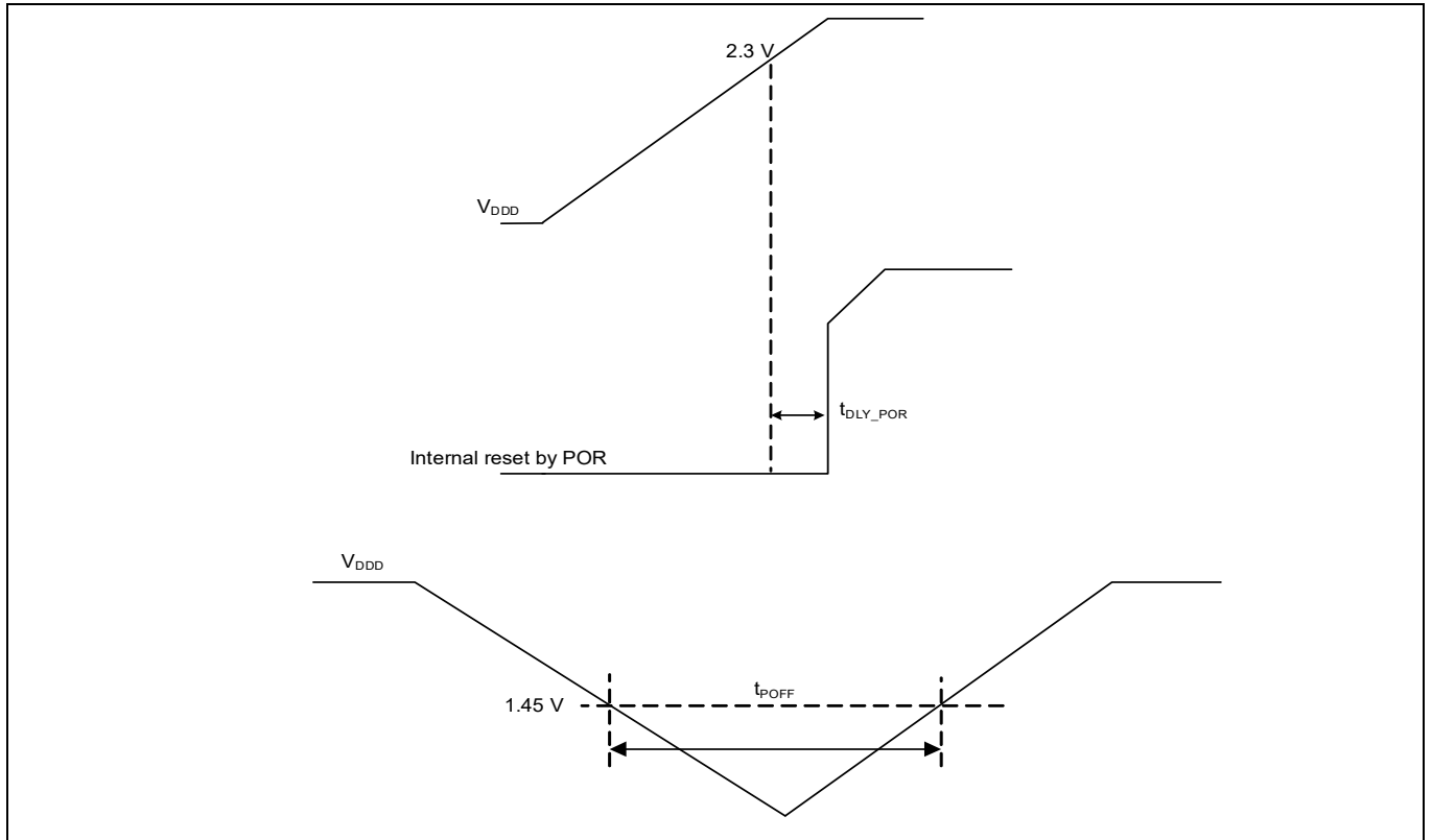
Figure 27-16 POR specifications
