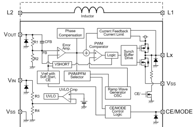
● XCL205 / XCL206 / XCL207 series B/C/G Type
