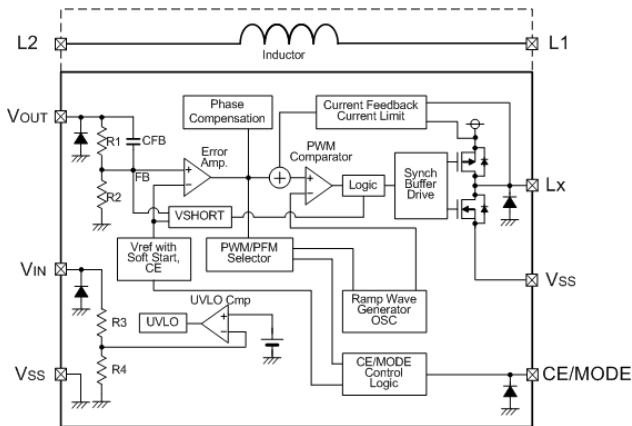
● XCL205 / XCL206 / XCL207 series A Type
