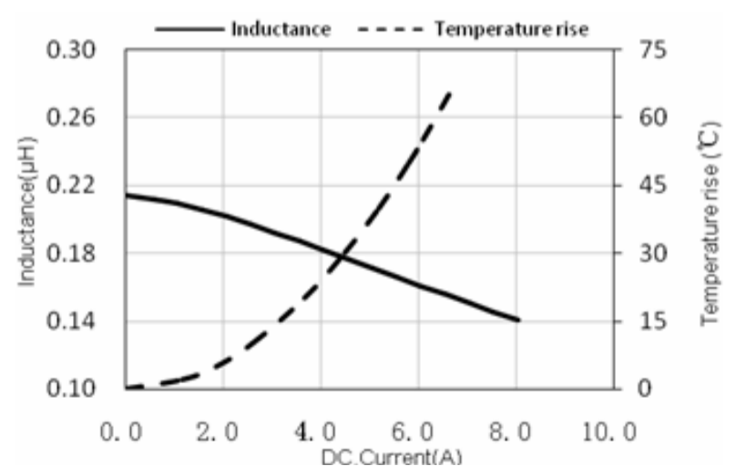
ASPI-U201610-R22
