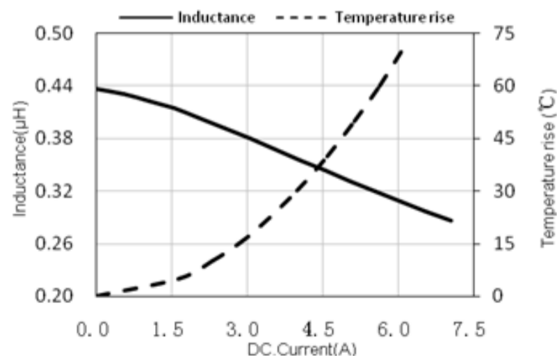
ASPI-U252010-R47
