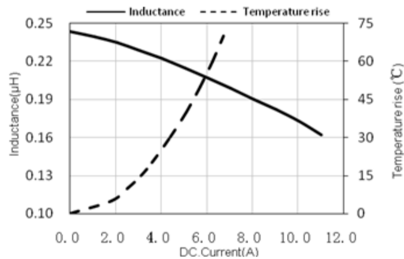
ASPI-U252010-R24
