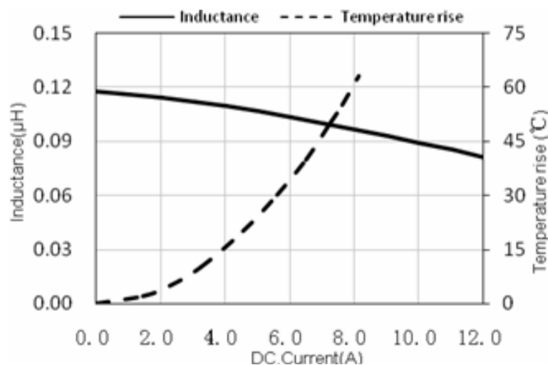
ASPI-U201610-R12
