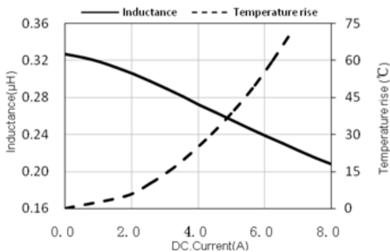
ASPI-U252010-R33
