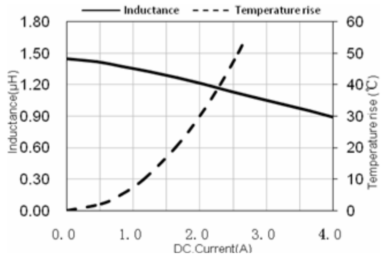
ASPI-U201610-1R5
