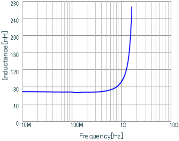
LQP03HQ68NJ02 L.
