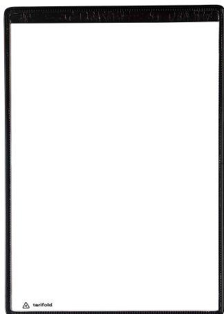
Poche magnétique
