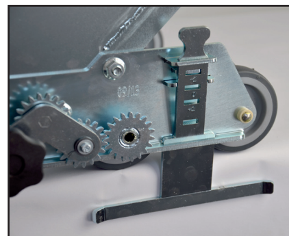
Seitenanschlag
