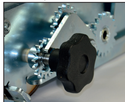
Handrad für Walzenfreilauf
