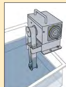
Typische Anwendung: Öl-Bandskimmer mit Montagefuß, montiert auf dem Rand eines Behälters
