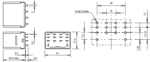
RH4V2-U/RH4V2-UL/RH4V2-UD
