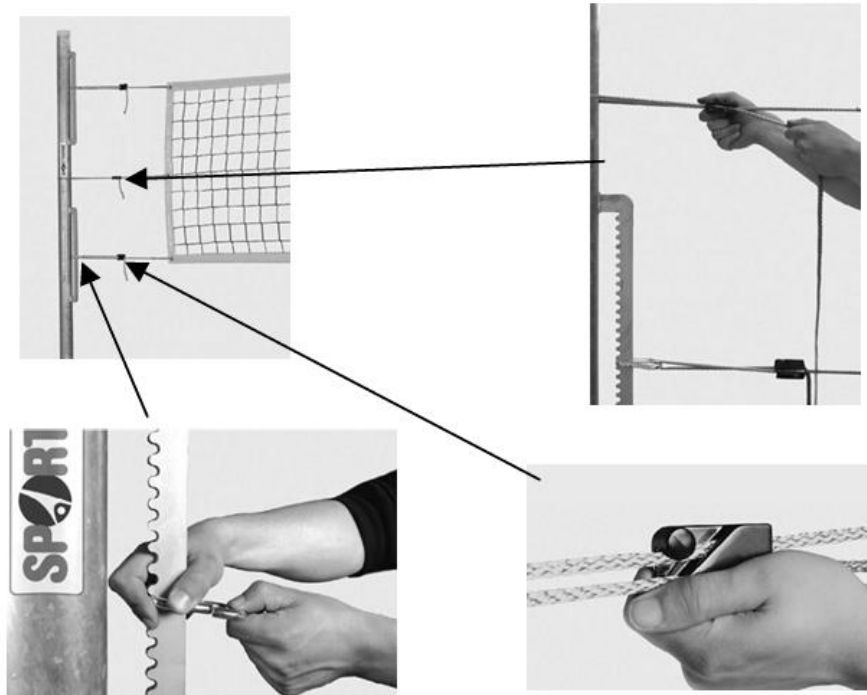
Abbildung 3: Netzbefestigung
