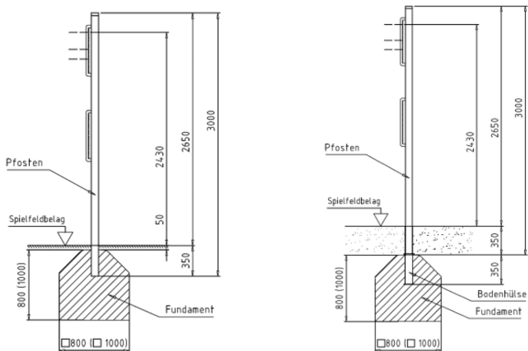
Abbildung 2: Fundament (ohne und mit Bodenlösung)
