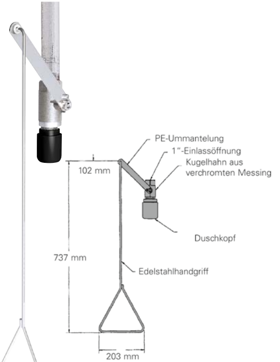
Körperdusche Typ G 1692 aus Edelstahl
