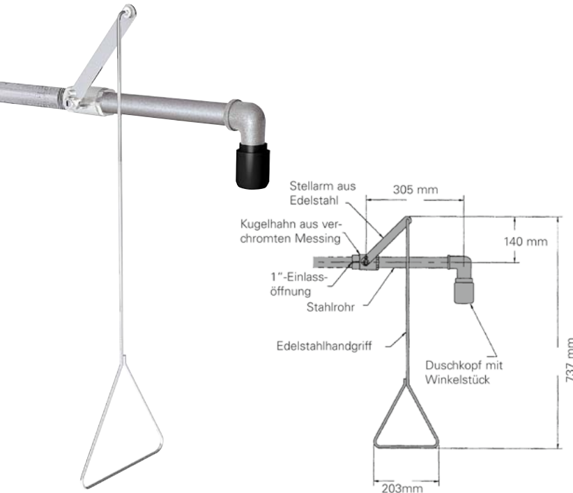
Körperdusche Typ G 1643, aus verzinktem Stahlrohr
