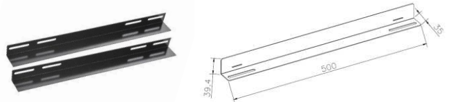
110-0169 Kit 2 rails Longueur 500mm
