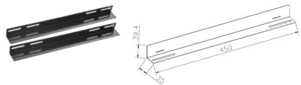
110-0186 Kit 2 rails Longueur 450mm
