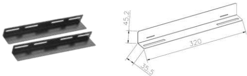
110-0185 Kit 2 rails Longueur 320mm
