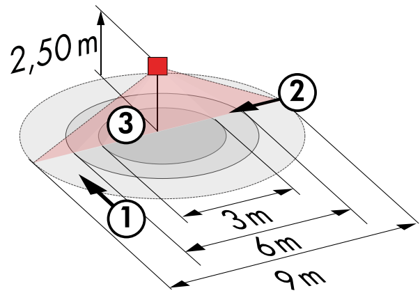
Reichweitendiagramm
