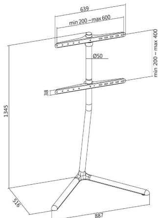
TV-Ständer, V-Fuß - Abmessungen
