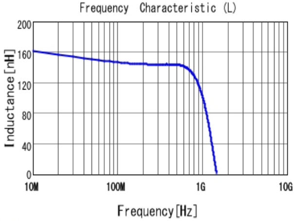
■ LQW18CAR16J00 L
