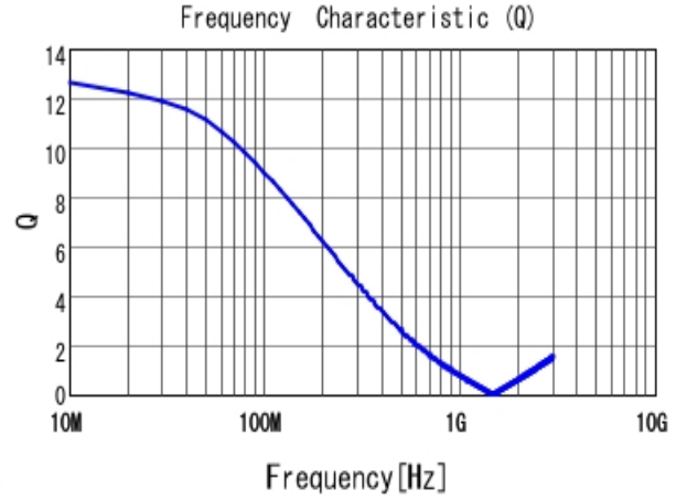
■ LQW18CAR16J00 Q
