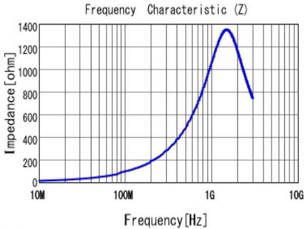
■ LQW18CAR16J00 |Z|
