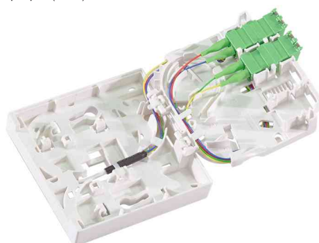
Visuel de référence : boîte d'épissure FTTH avec câble de pose, 2x LCD / APC
