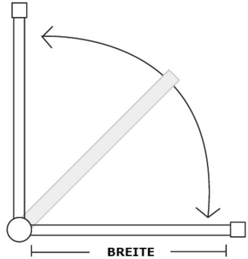
Technische Ansicht: Drehschranke, beschichtet, mit Dreikant und Bodenplatte (Art. 413.250v)
