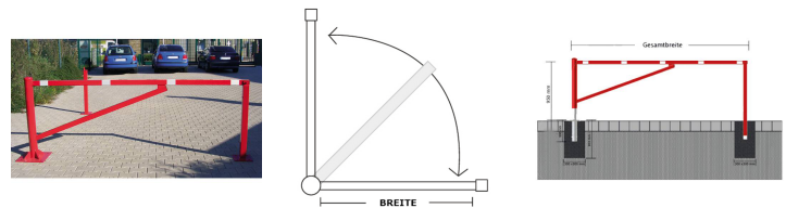
Modellbeispiel: Drehschranke beschichtet mit Dreikant und Bodenplatte (Art. 413.250bfp)
