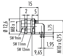
Leiterplattendicke: 1,6 mm
