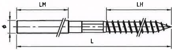
Stockschraube Standard Sechskant zwischen dem Gewinde. Durchmesser(φ) M6, M8, M10, M12
