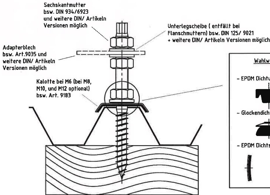
Stockschraube Standard Sechskant zwischen dem Gewinde. Durchmesser(φ) M6, M8, M10, M12
