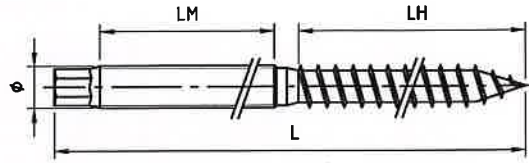
Stockschraube mit Aussensechskant. Durchmesser(φ) M10 und M12
