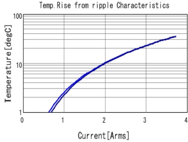
GRM155R61A475MEAA Temp. rise ■ 500kHz ■ 1MHz
