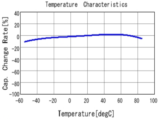
■ GRM155R61A475MEAA C-Temp. capchange, DCO. 0V, ACO. 1V rm
