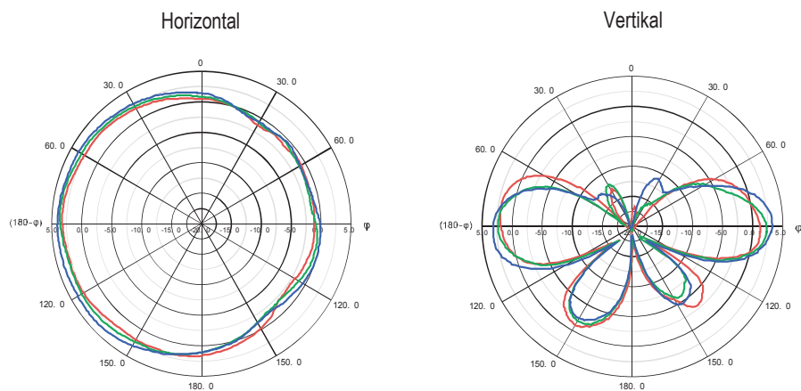
Strahlungsdiagramm 2,4 GHz
