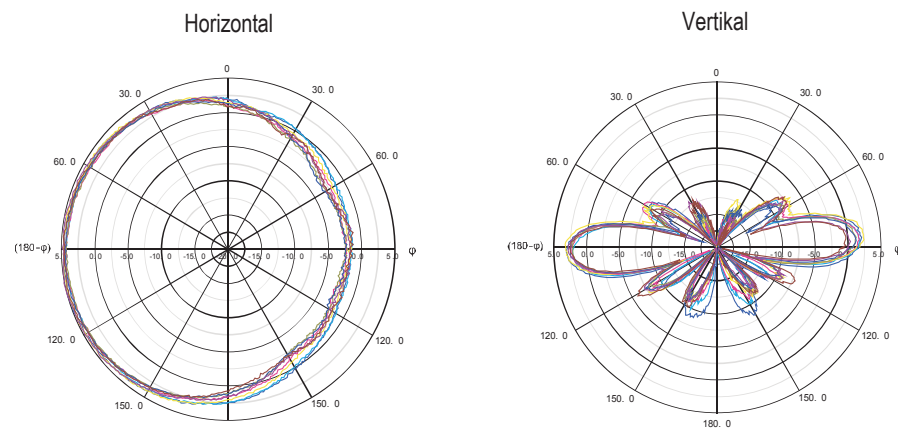
Strahlungsdiagramm 5 GHz
