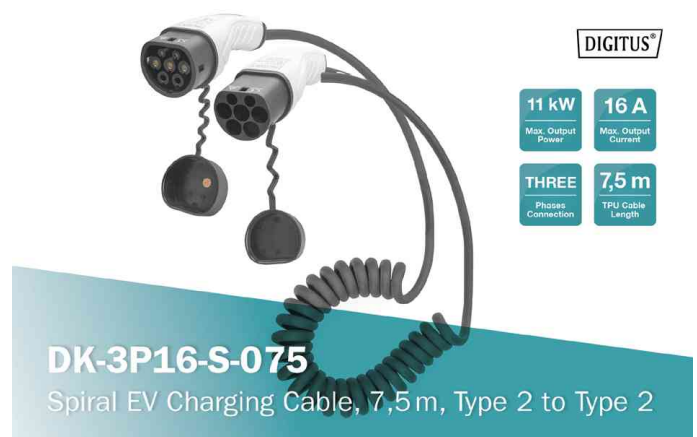
E-Auto-Ladekabel, Typ 2, 3-phasig, Detailansicht Stecker
