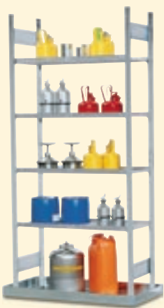
Gefahrstoffregal Typ GRB 1060
