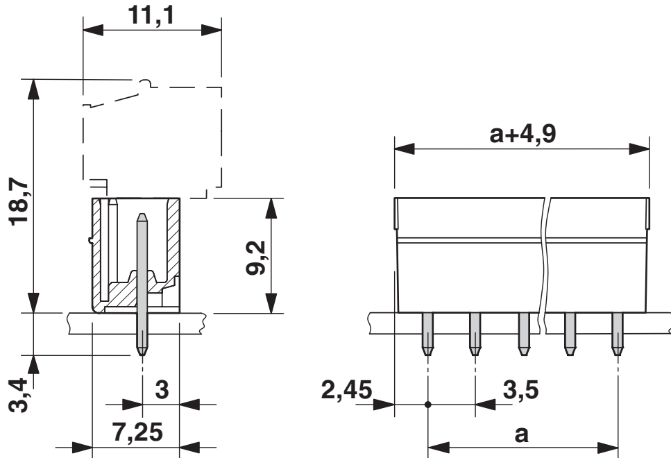
Maßzeichnung
