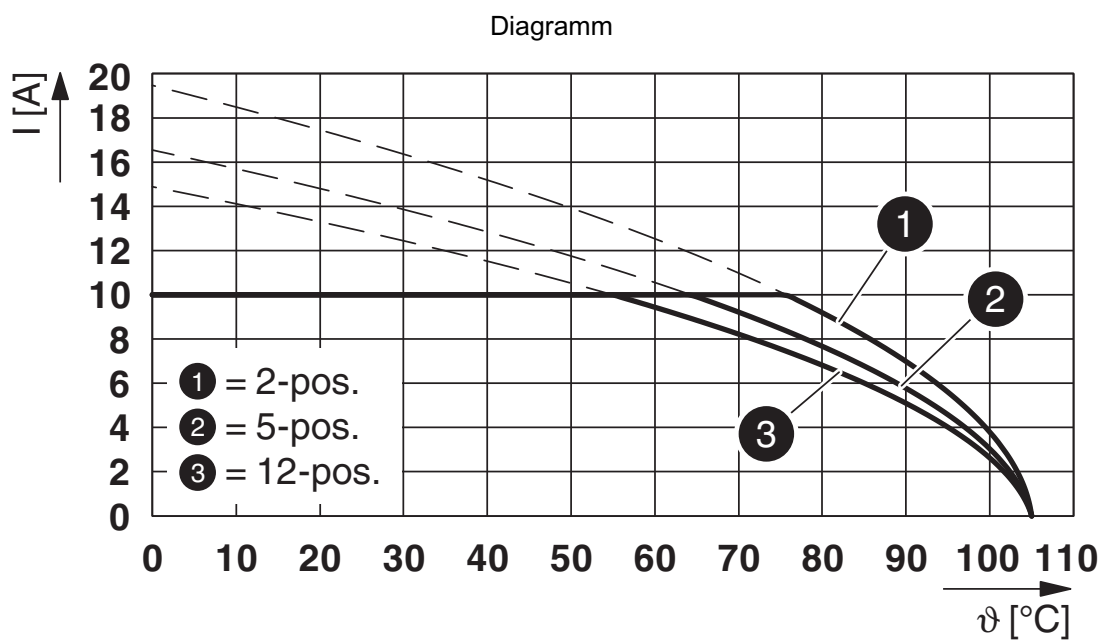
Typ: FKCVW 2,5/...-STF mit MDSTBV 2,5/...-GF
