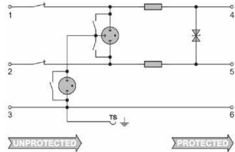
Prinzipschaltbild
