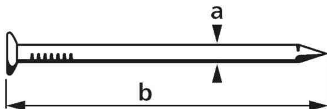
Visuel de référence: pointe, tête fraisée, pictogramme
