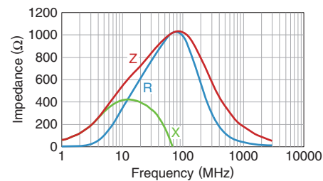
MMZ1608R102ATD25
