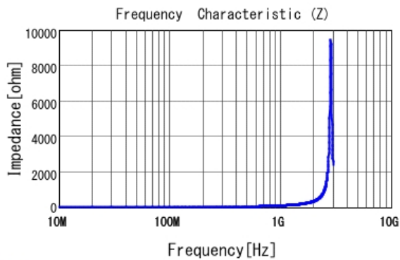
■ LQG15HH15NJ02 |Z|
