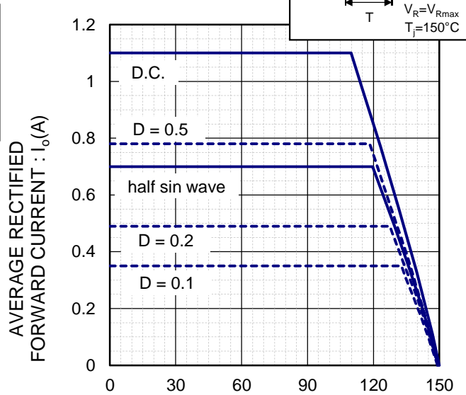
LEAD TEMPERATURE : T_l (°C) DERATING CURVE ( I_o - T_l )
